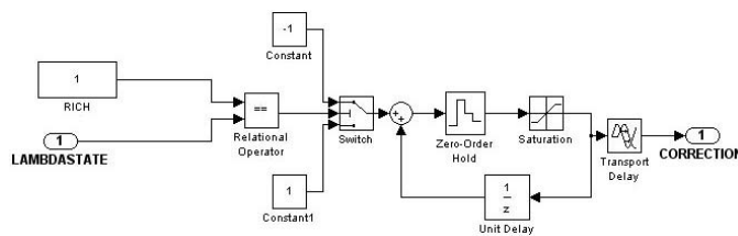
Fig. 4. GTIT control algorithm.
