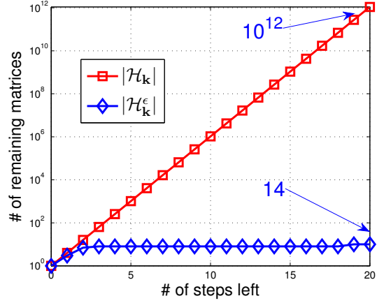
Fig. 2. Evolution of |\mathcal{H}_k^\epsilon|
