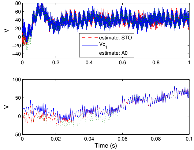
Fig. 2. v_{c_1} (—), \hat{v}_{c_1} , STO (- - -) and AO (...).
