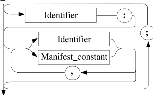
Parent_list
