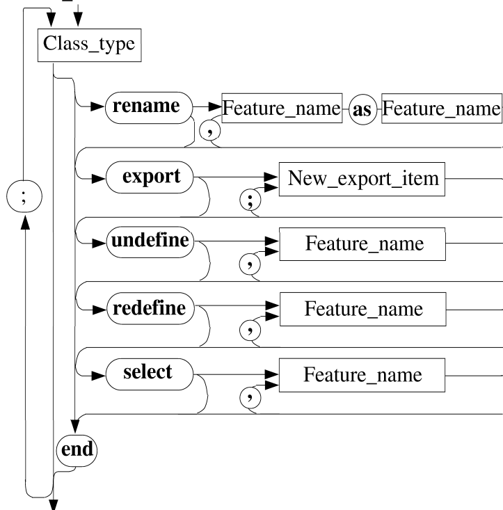
Parent_list
